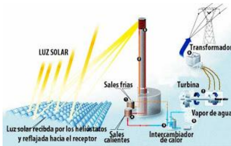
Esquema de funcionamiento Planta termosolar con sistema de acumulación de calor. Fuente: manuelricosecades.blogspot.com
