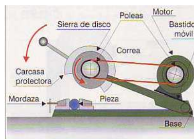
Figura 12.6. Esquema de una sierra de disco.
