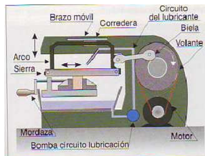
Figura 12.4a. Sierra mecánica de movimiento lineal alternativo.
