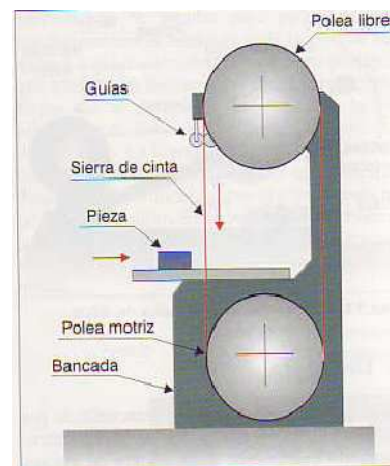
Figura 12.5a. Esquema de una sierra de cinta.
